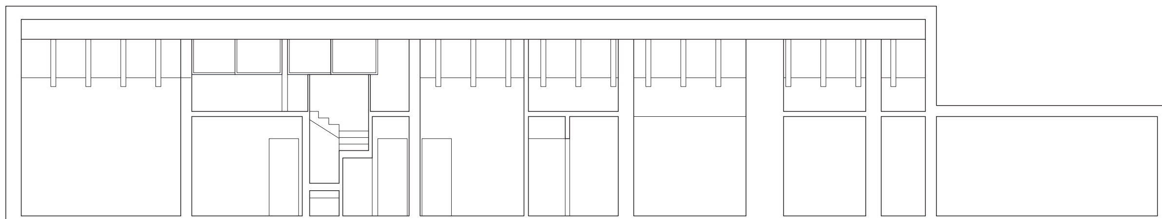
SEZIONE A-A
