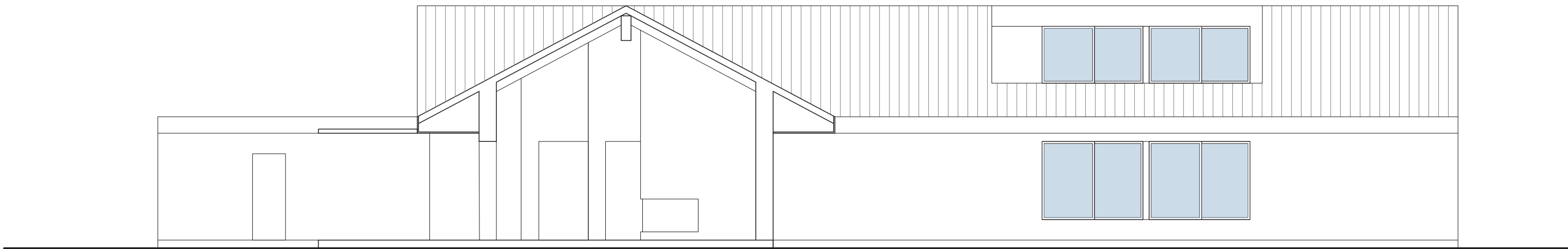
SEZIONE E-E
